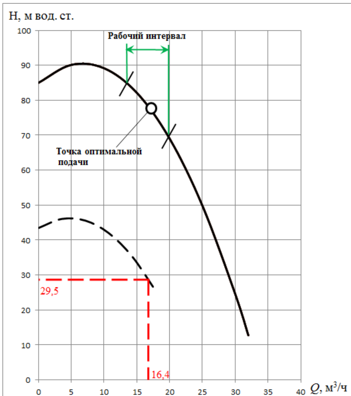
Рисунок 6.1 – Анализ характеристики насоса, установленного в скважине № 68-Г
