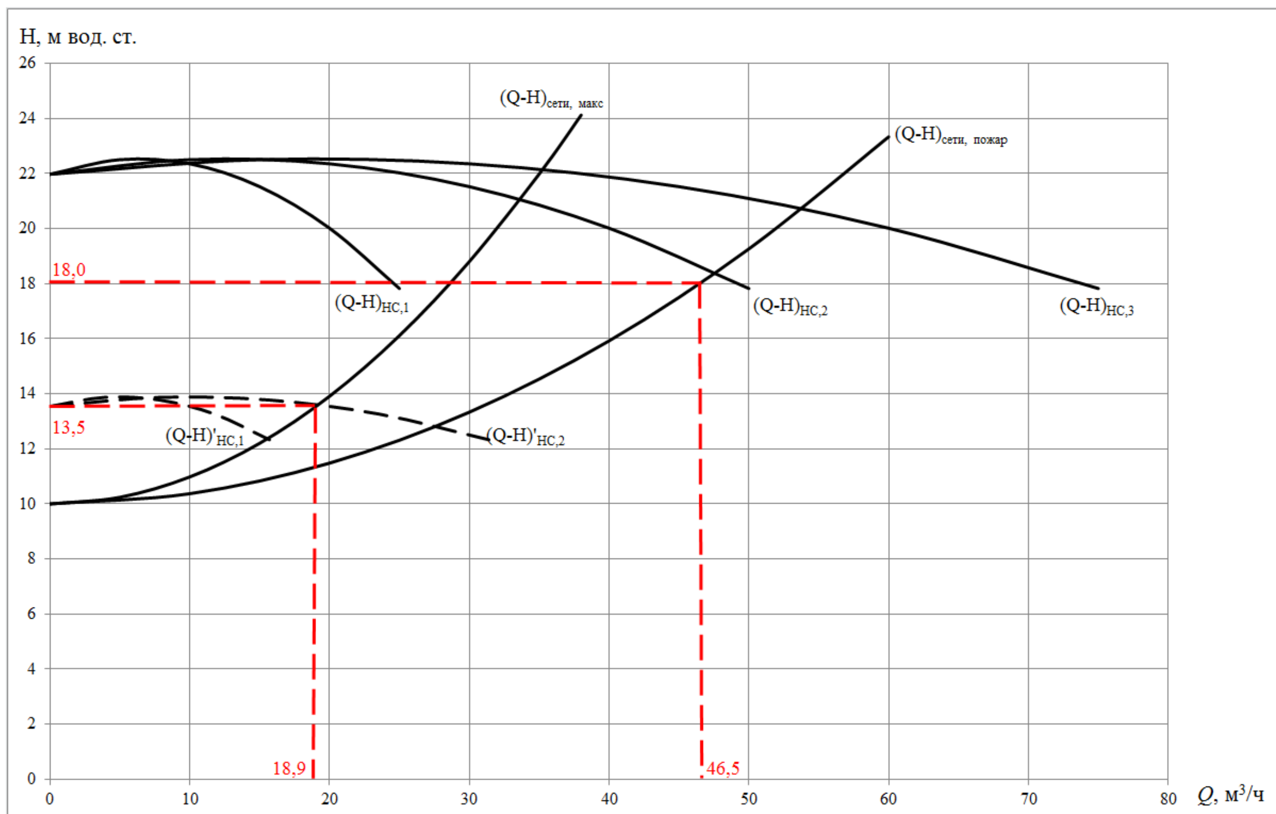
Рисунок 6.2 – Совмещенные расходно-напорные характеристики насосов и водопроводной сети при расчетных режимах работы сети
