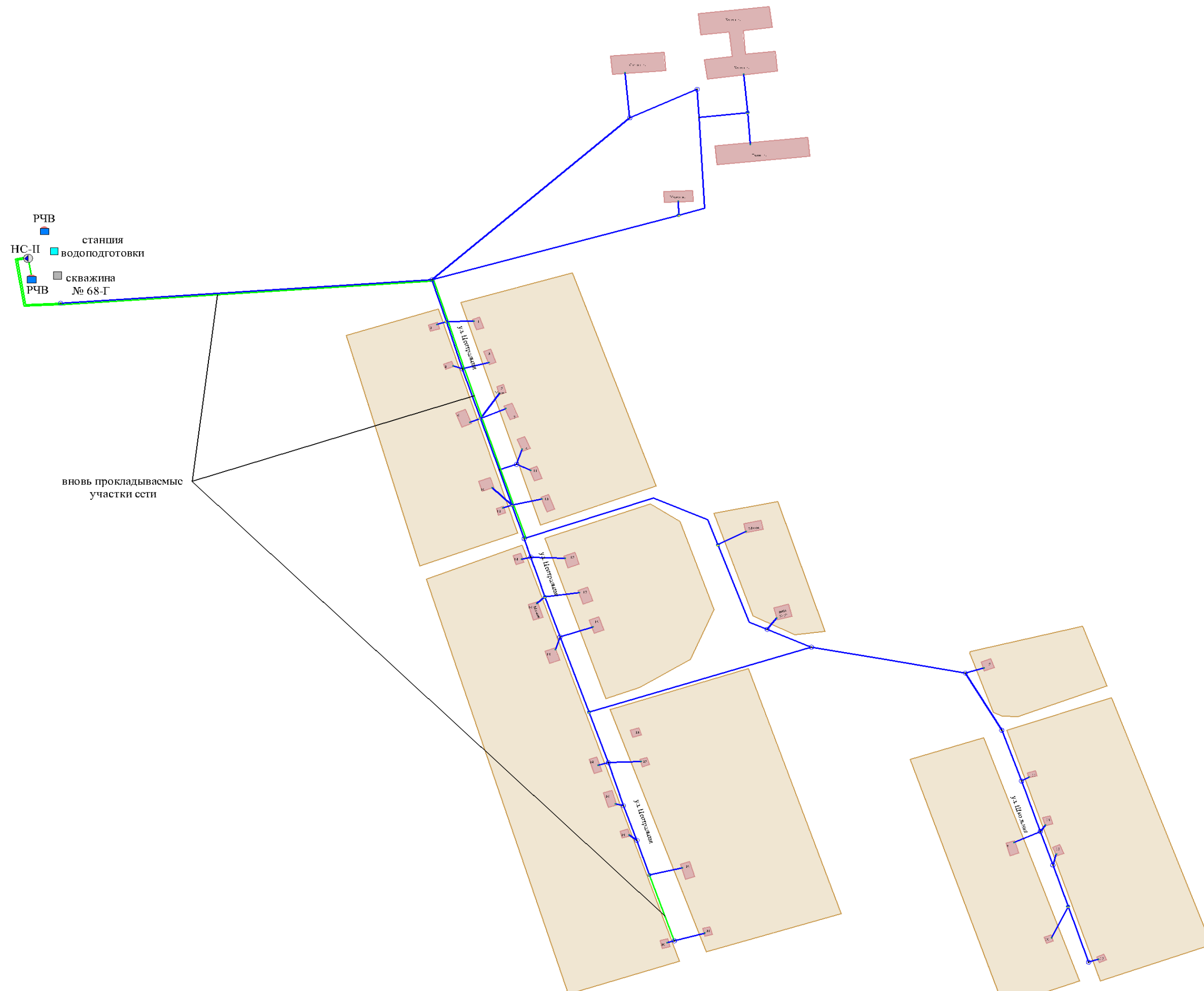
Рисунок 6.4 – Схема планируемого размещения объектов централизованной системы водоснабжения
