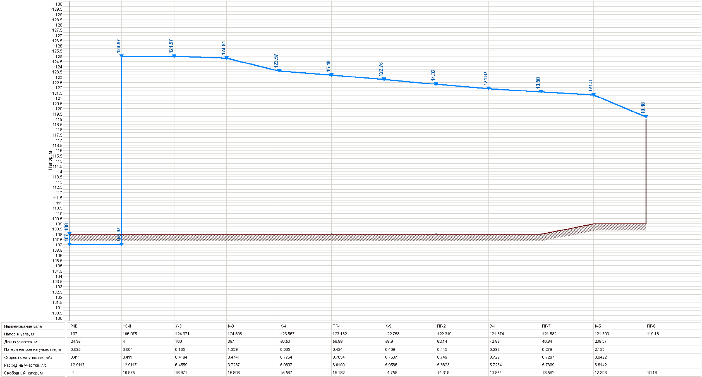
Рисунок 3.11 – Пьезометрический график от резервуаров чистой воды до пожарного гидранта ПГ-6 для режима пожаротушения
