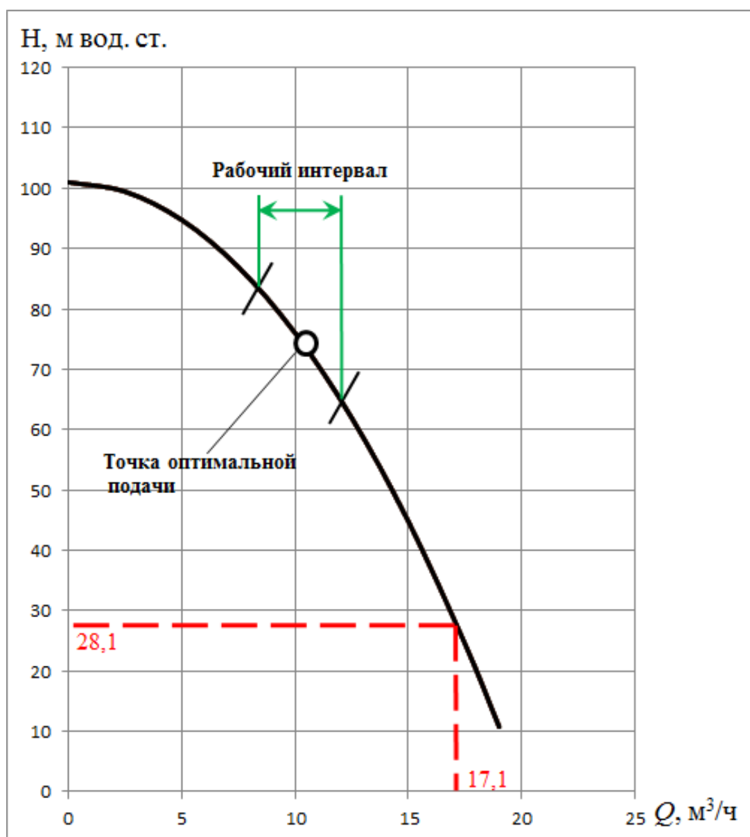
Рисунок 6.1 – Анализ характеристики насоса, установленного в скважине № ОМ-189
