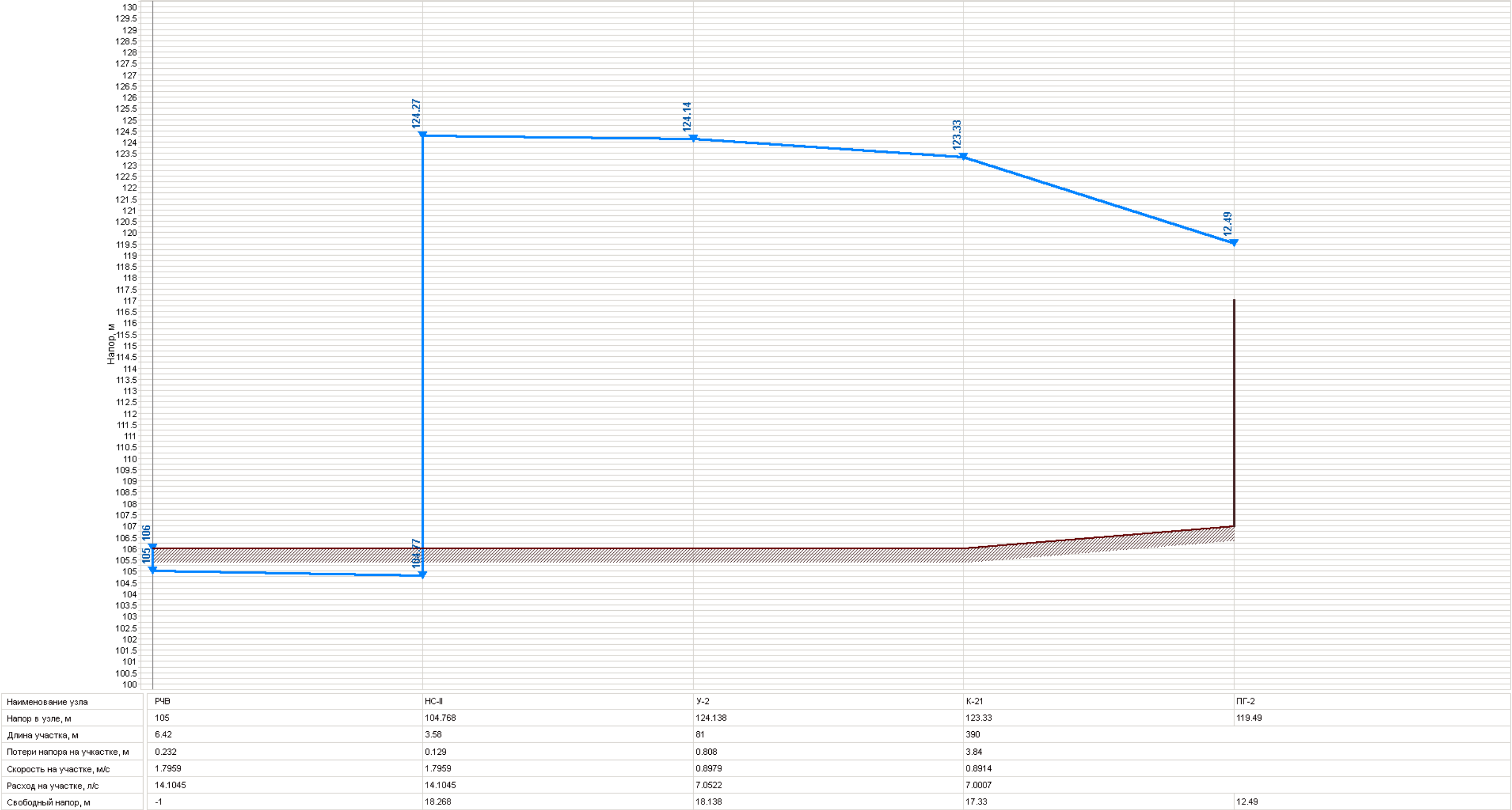
Рисунок 3.11 – Пьезометрический график от резервуаров чистой воды до пожарного гидранта ПГ-2 для режима пожаротушения
