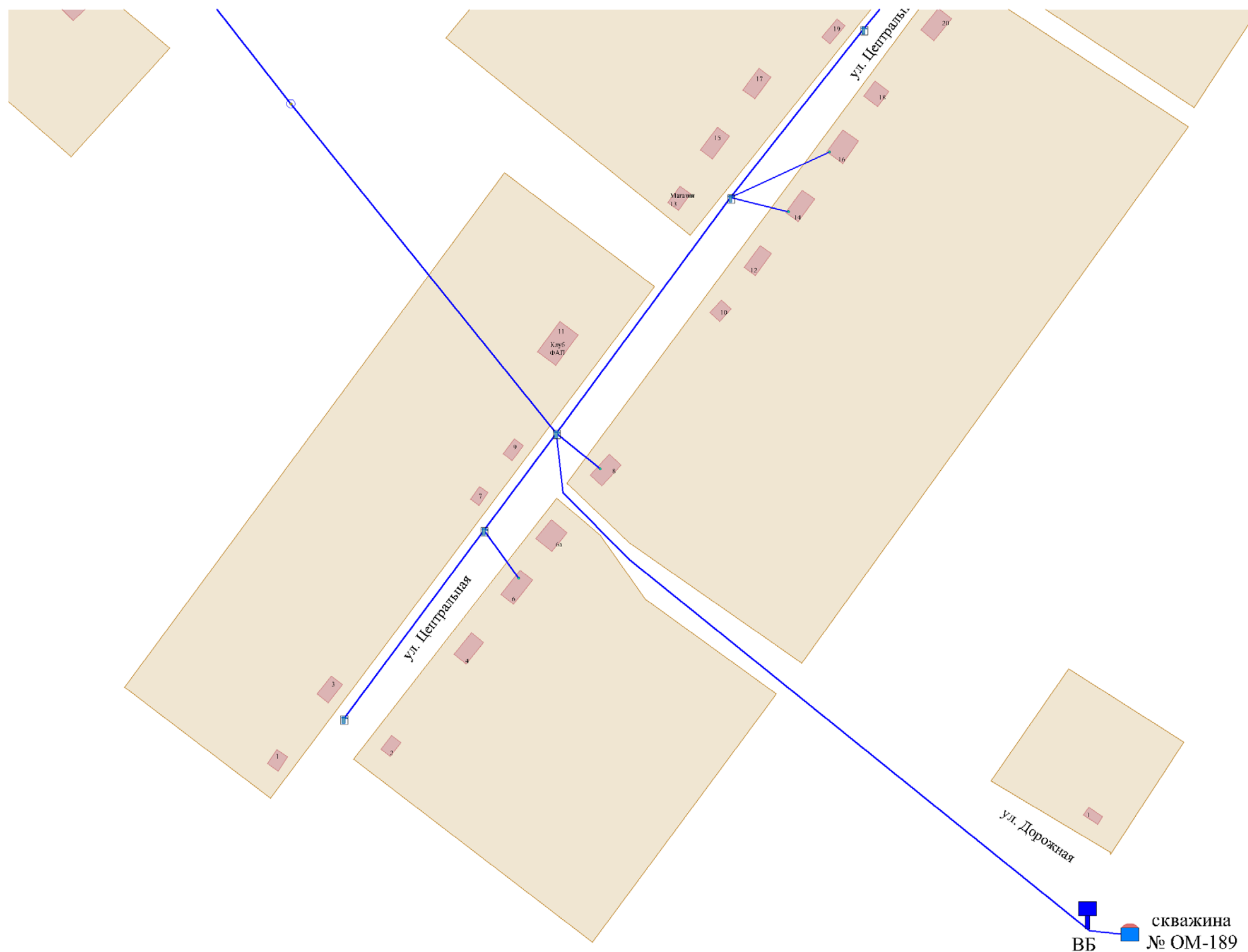
Рисунок 6.3 – Схема существующего размещения объектов централизованной системы водоснабжения
