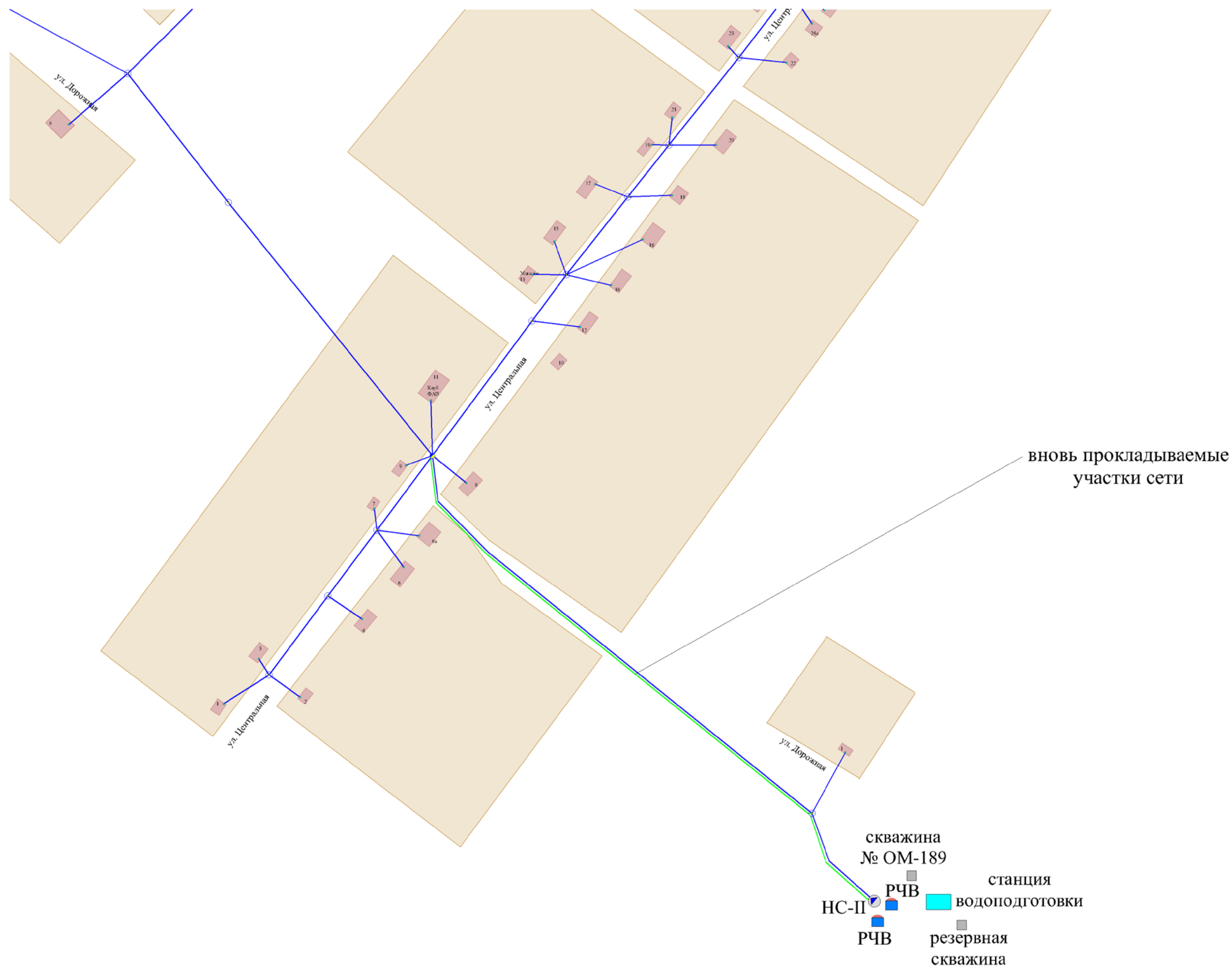
Рисунок 6.4 – Схема планируемого размещения объектов централизованной системы водоснабжения
