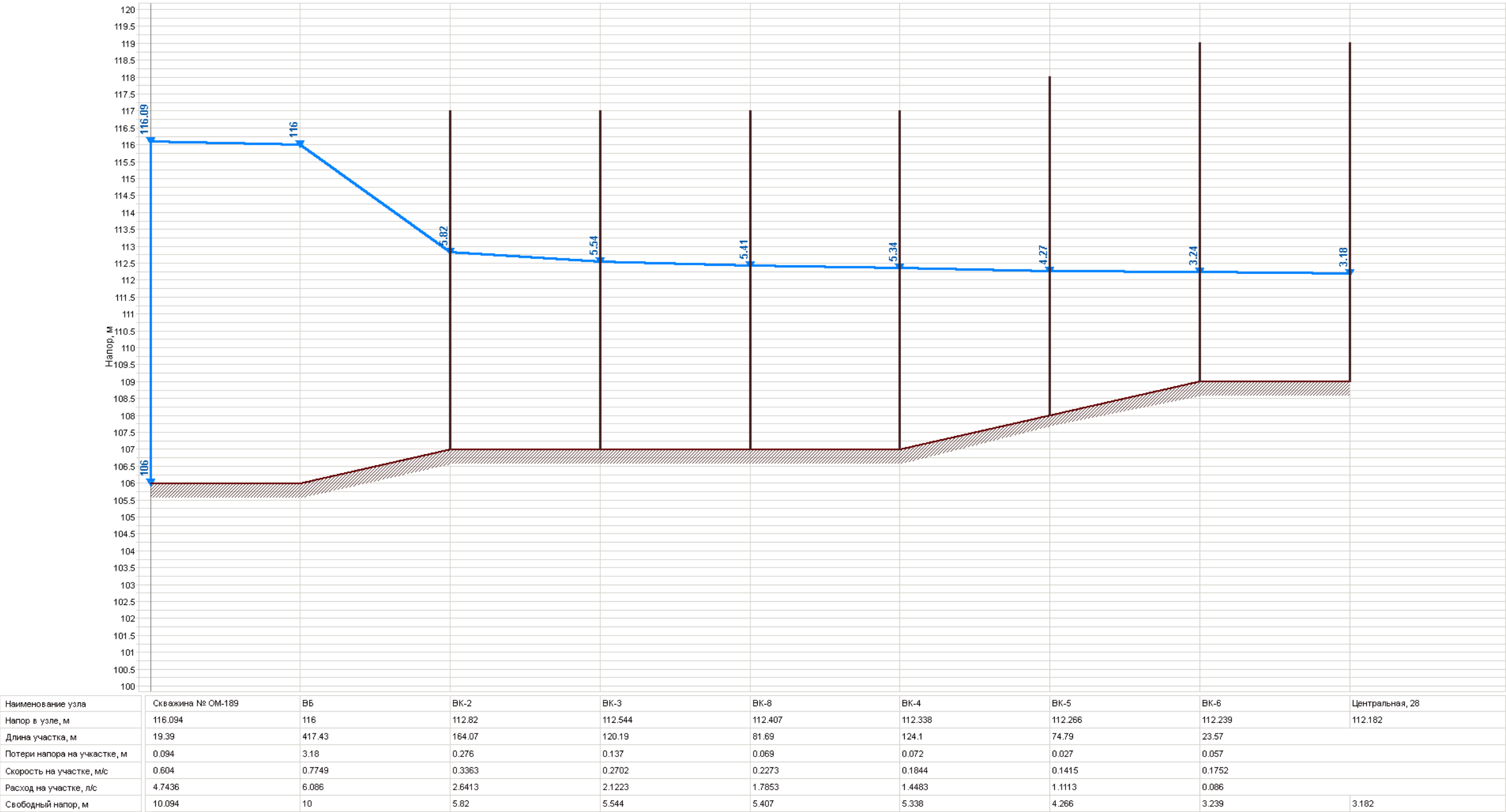
Рисунок 3.9 – Пьезометрический график от водозаборной скважины до диктующего потребителя
